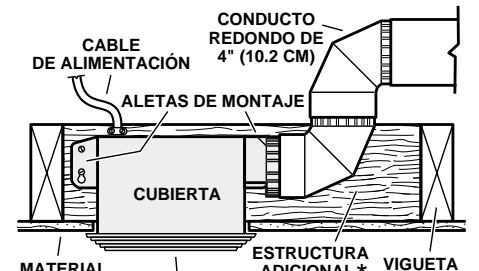
CUBIERTA MONTADA EN UNA ESTRUCTURA ADICIONAL Descarga a 90° de las viguetas.
